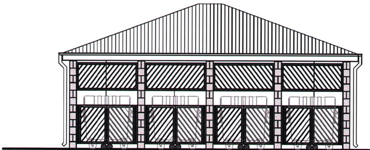
ELEWACJA WSCHODNIA
